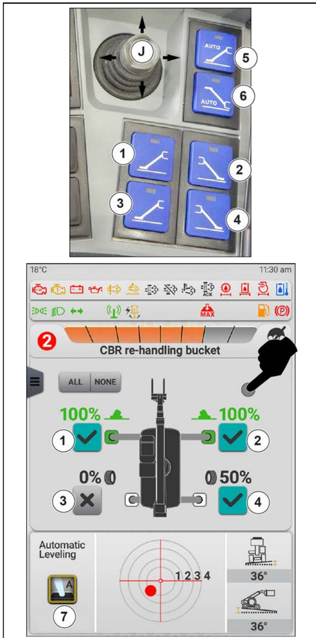
Afbeelding 135: Handmatige stabilisatieprocedure
