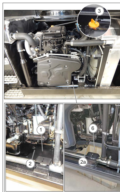
Afbeelding 179: Motorolie aftappen
