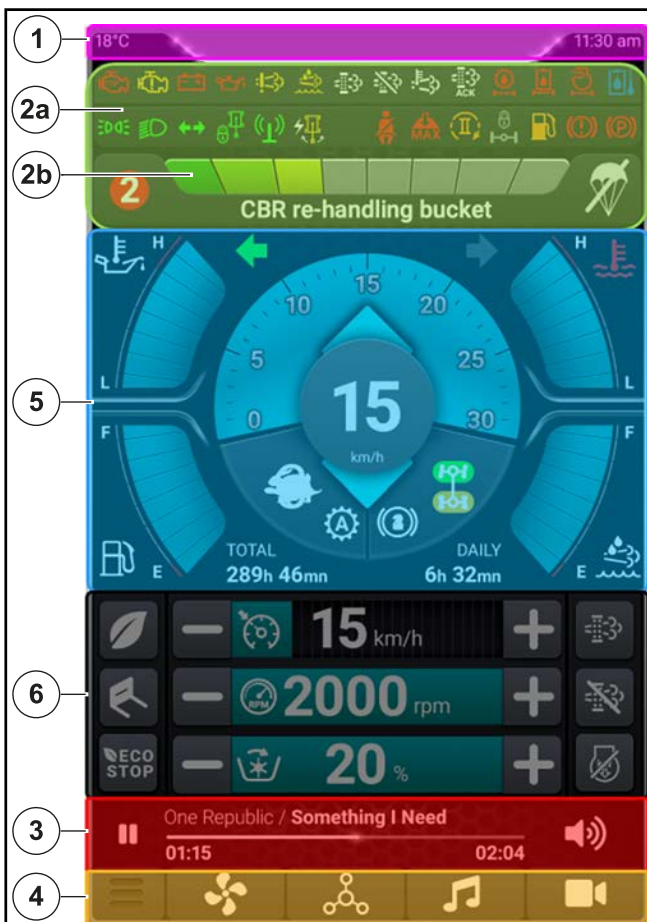
Afbeelding 78: HMI-gebied
