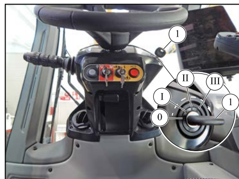
Afbeelding 73: Contactschakelaar
