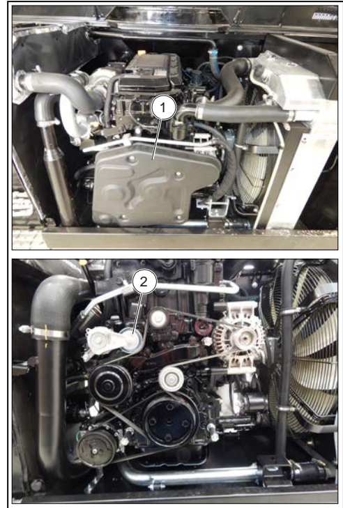
Afbelding 208: De servicieriem van de driefasemotor vervangen
