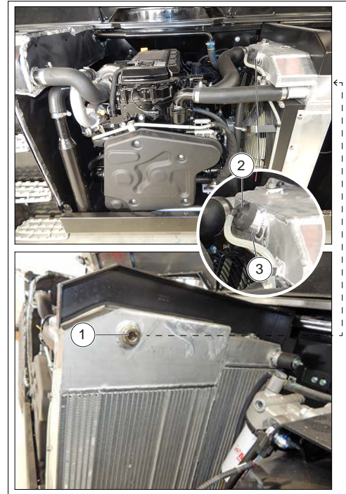
Afbeelding 145: Koelvloeistofpeil
