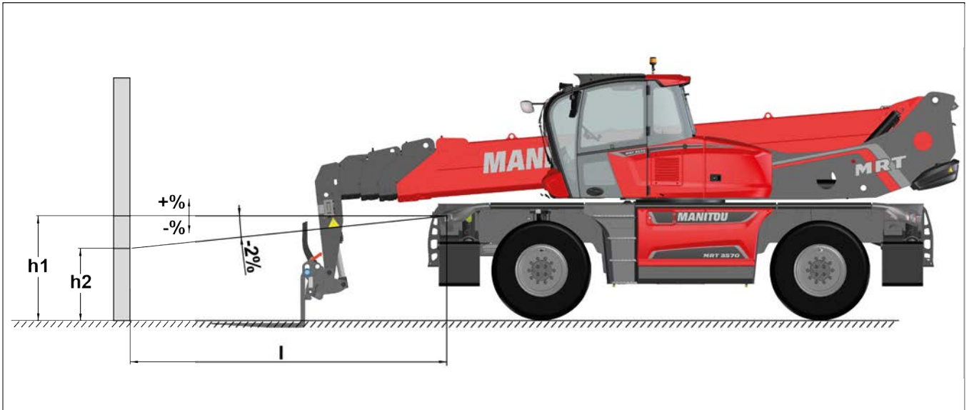
Afbeelding 213: De koplampen afstellen
