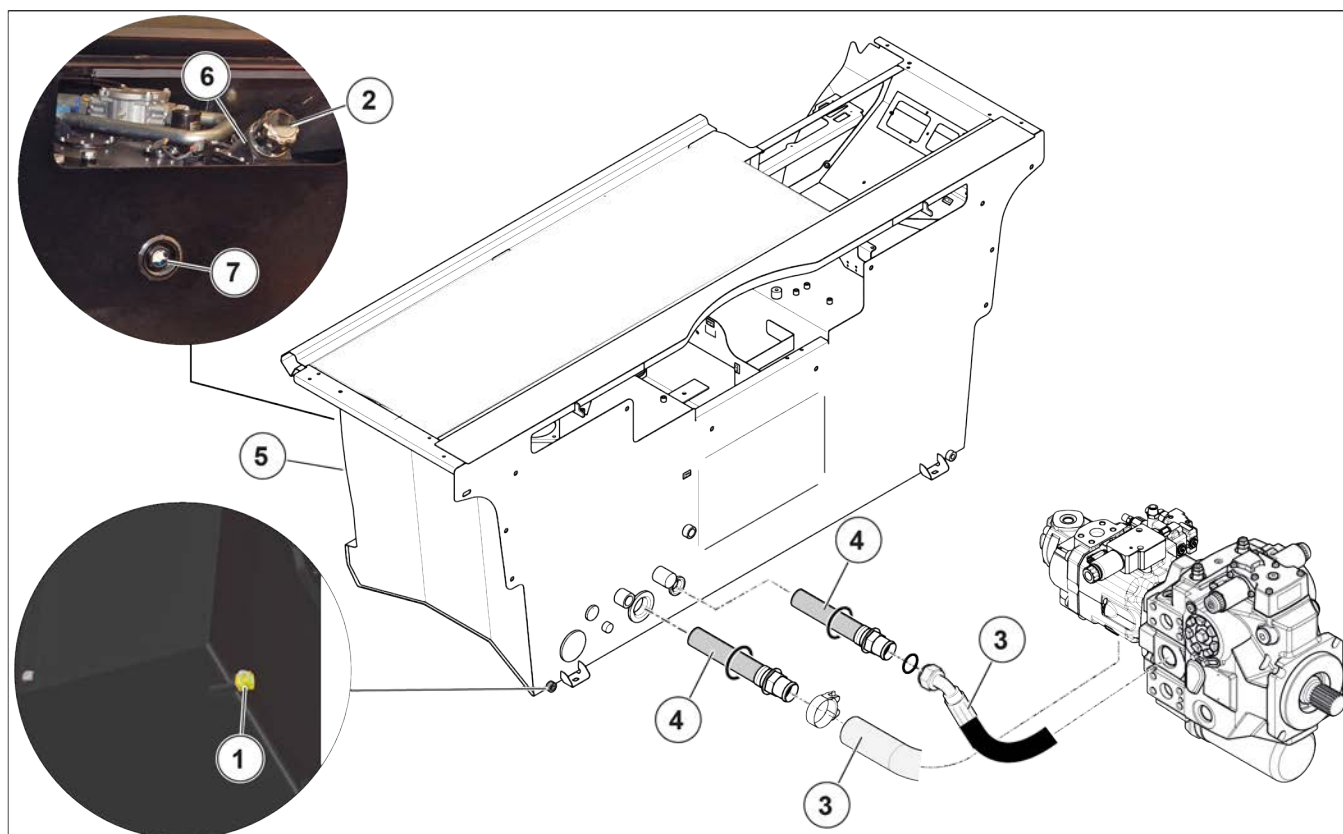
Afbeelding 206: De hydraulische olie verversen en de filterpatroon van het inlaatfilter van de hydraulica reinigen
