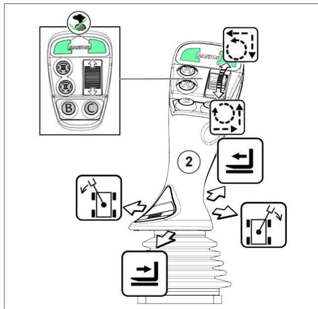
Afbeelding 103: Joystick links
