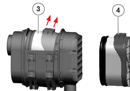
Afbeelding 186: Patroon drogeluchtfilter vervangen 8492801-LE-EMC(A/2021)
