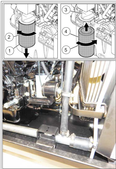
Afbeelding 180: Motoroliefilter vervangen
